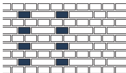
Holländischer Verband
