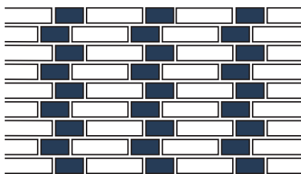
Gotischer Verband
