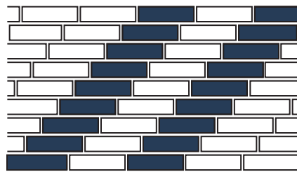
Läuferverband 1/4 Stein schräg versetzt
