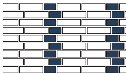
Schlesischer Verband
