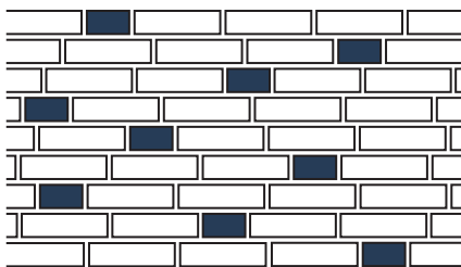
Wilder Verband
