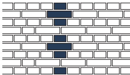
Kreuzverband
