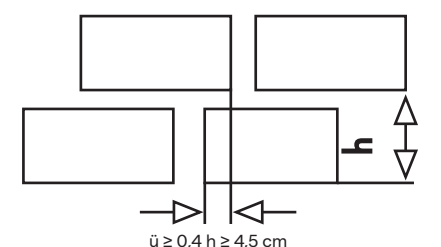
Läuferverband 1/4 Stein senkrecht versetzt
