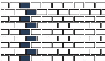
Kopfverband
