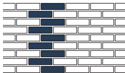
Läuferverband 1/2 Stein versetzt
