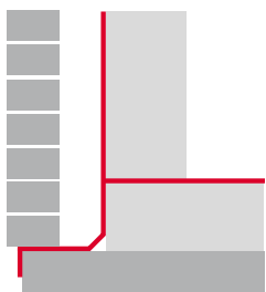
Prinzip Sockelabdichtung
