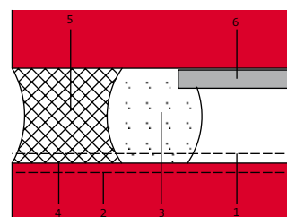
Dehnungsfuge Ausbildung vertikal und horizontal:
