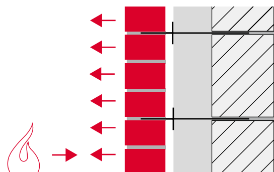
Brandschutz
