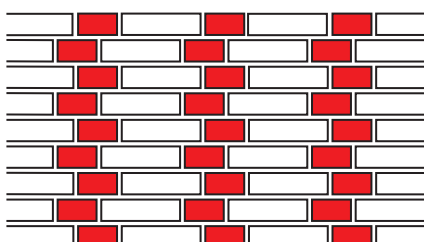
Gotischer Verband
