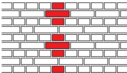
Kreuzverband
