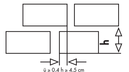
Überbindemaß, bezogen auf die Klinkerhöhe
