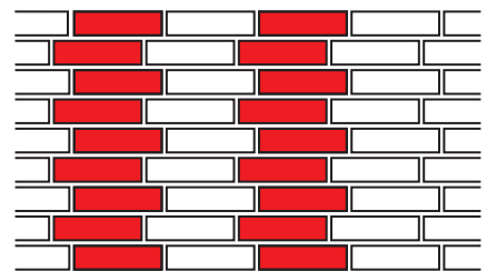
Läuferverband 1/4 Stein senkrecht versetzt
