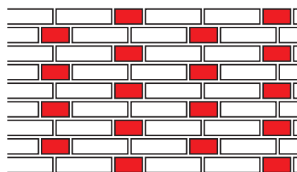
Märkischer Verband
